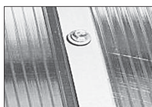
Усиленное крепление: саморез + оцинкованная лента.
